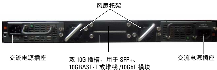
图 1-10. PC7048R 背面板
